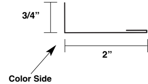
J Trim VTJT
