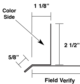
Header/Jamb Base Trim VTHJB
