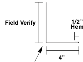
Jamb Trim MT-179
