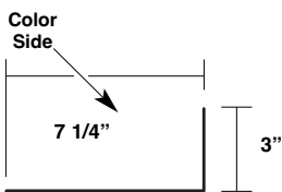
Rake Tie-In Trim Item #: 38432
