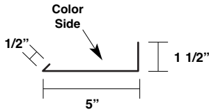
Flared Edge Trim Item #: 38383
