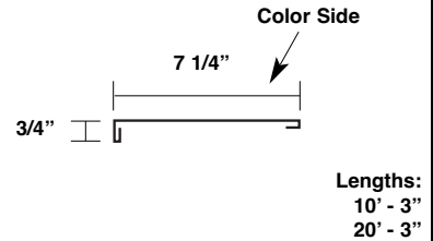
Rake End ML-RE
