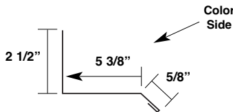
Rake Tie-In
