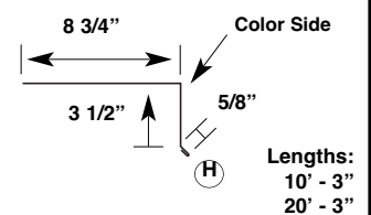
High Side Trim* M2HS
