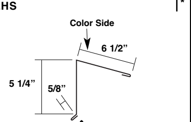
Hi-Side Trim* MDLHS
