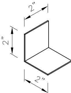
CLIP 16 GA.
