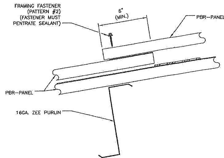
DETAIL A1
