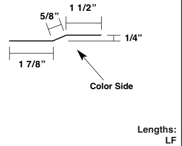
Rake Trim MT-183
