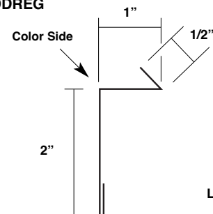
Reglet MODREG
