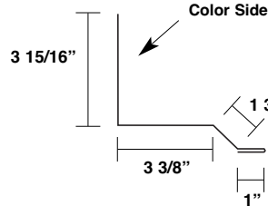
Step Rake Tie-In MODSEW
