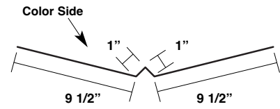
Valley Trim* MODVT
