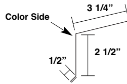
Denver Eave Trim* MODDE
