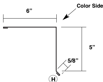
Rake Trim MT-183
