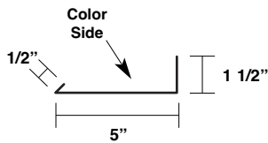
Contoured Eave Trim*
