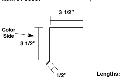
Valley Pan Trim*
