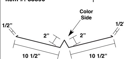
Valley Pan Trim*
