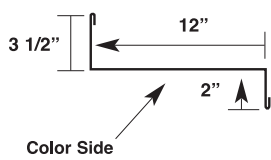
Valley Trim* (P-VF)
