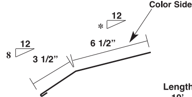
Gambrel Upper* (P-GU)
