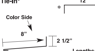
Ridge Trim* (R-RF)
