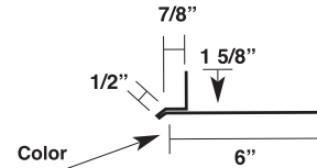
Overhead Door Drip 6" (P-ODP-6)
