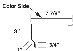
Overhead Door Flashing-A (P-JF-A)
