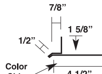
Overhead Door Drip 4 1/2" (P-ODP-4 1/2)
