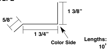
Rake Trim MDLRT
